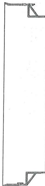
承口示意图
