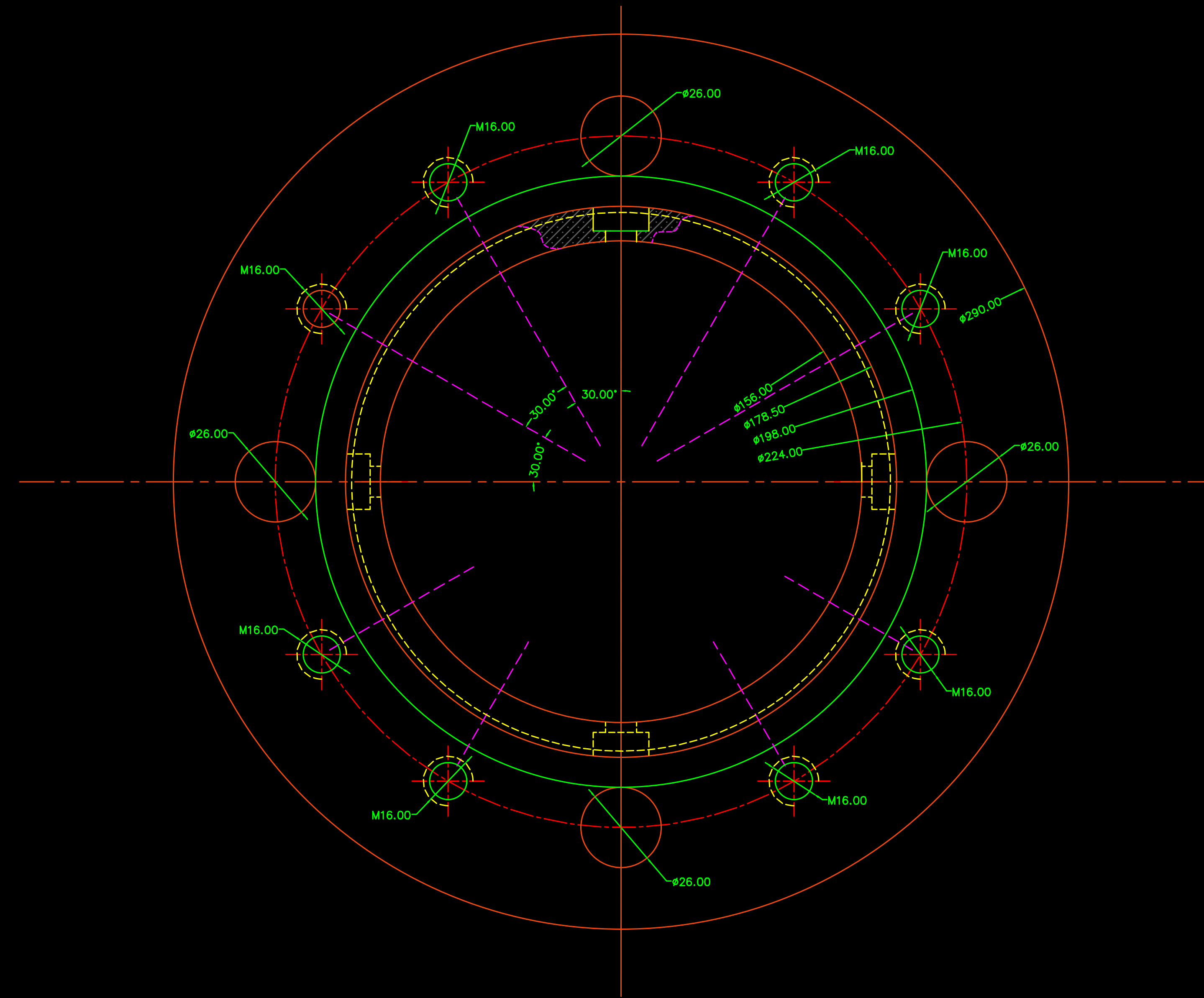
左视图
