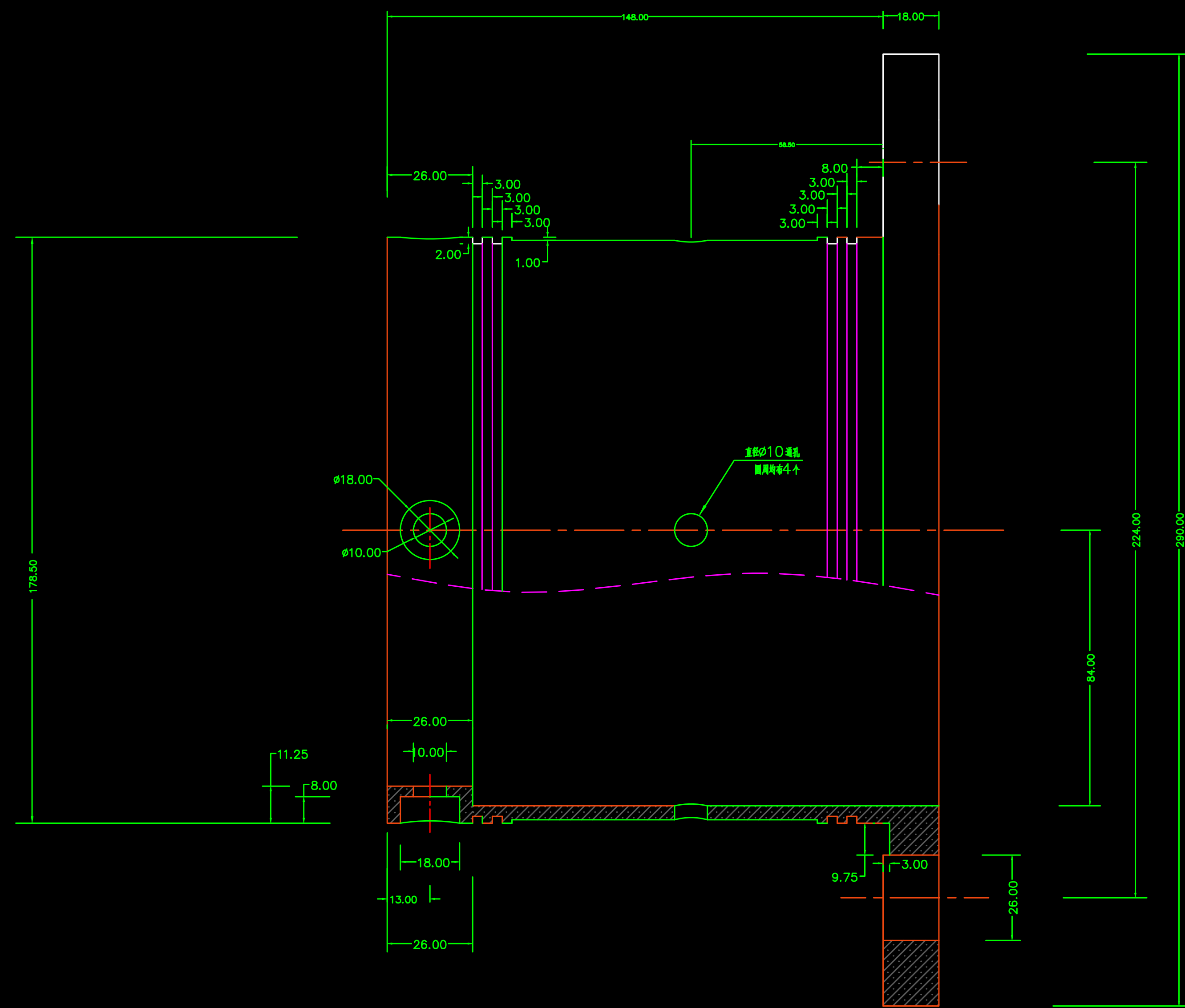
正视图
