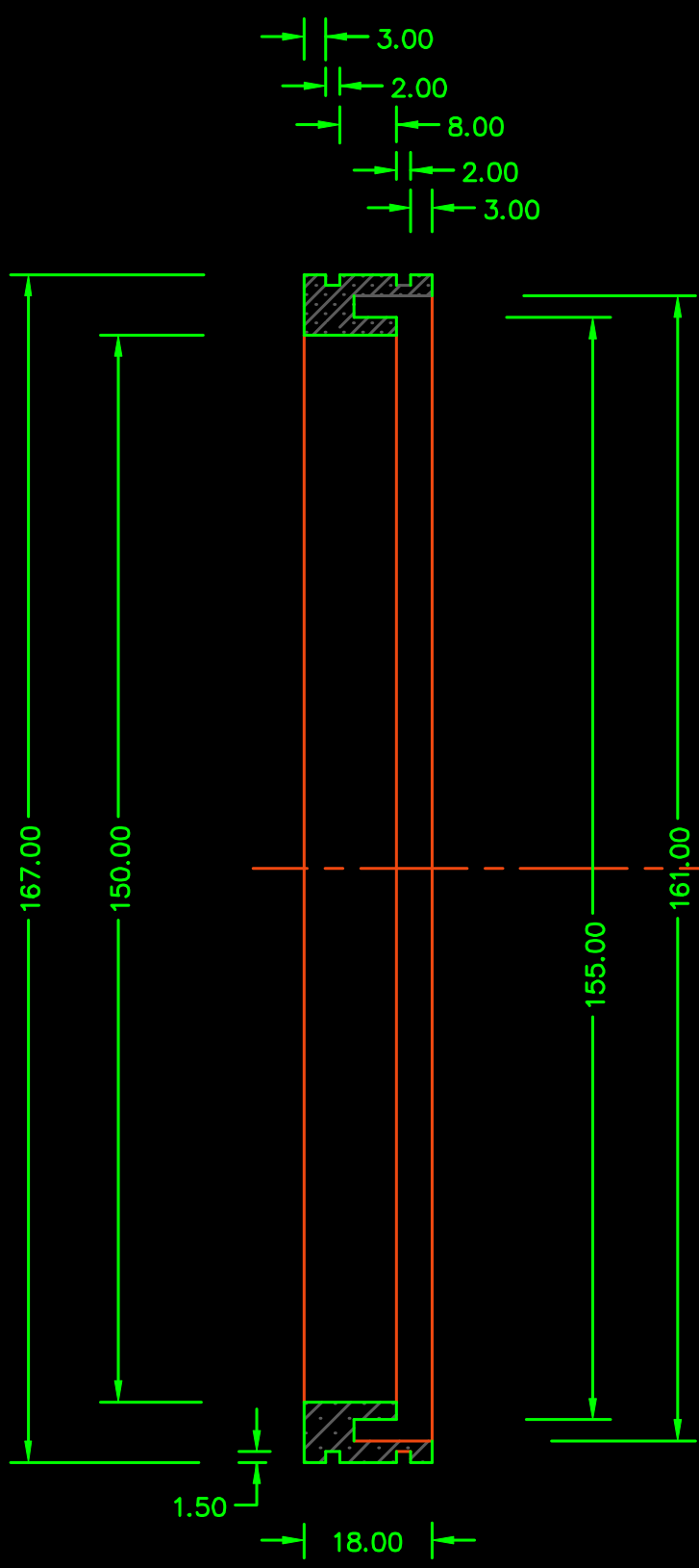
正视图
