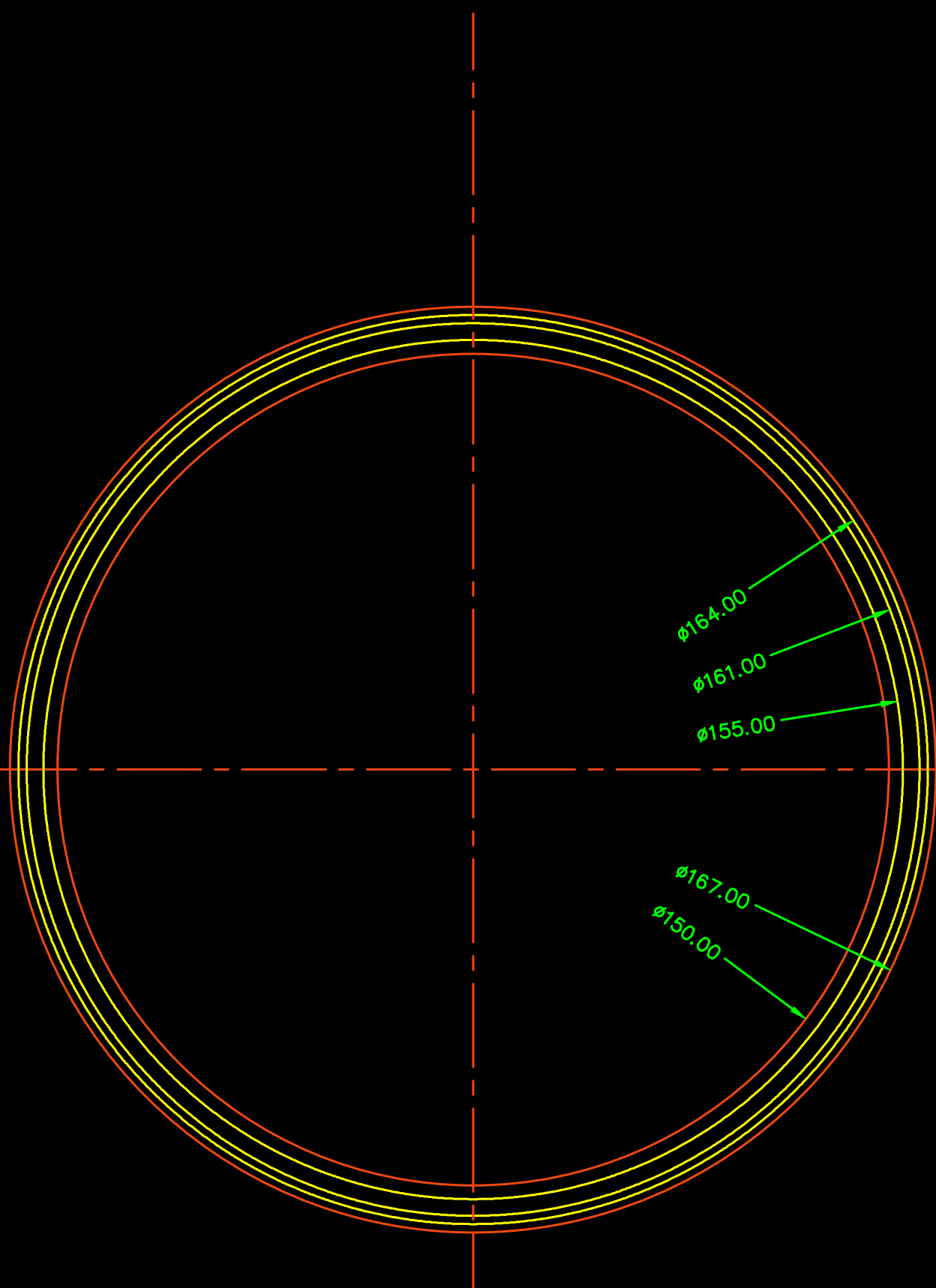
左视图
