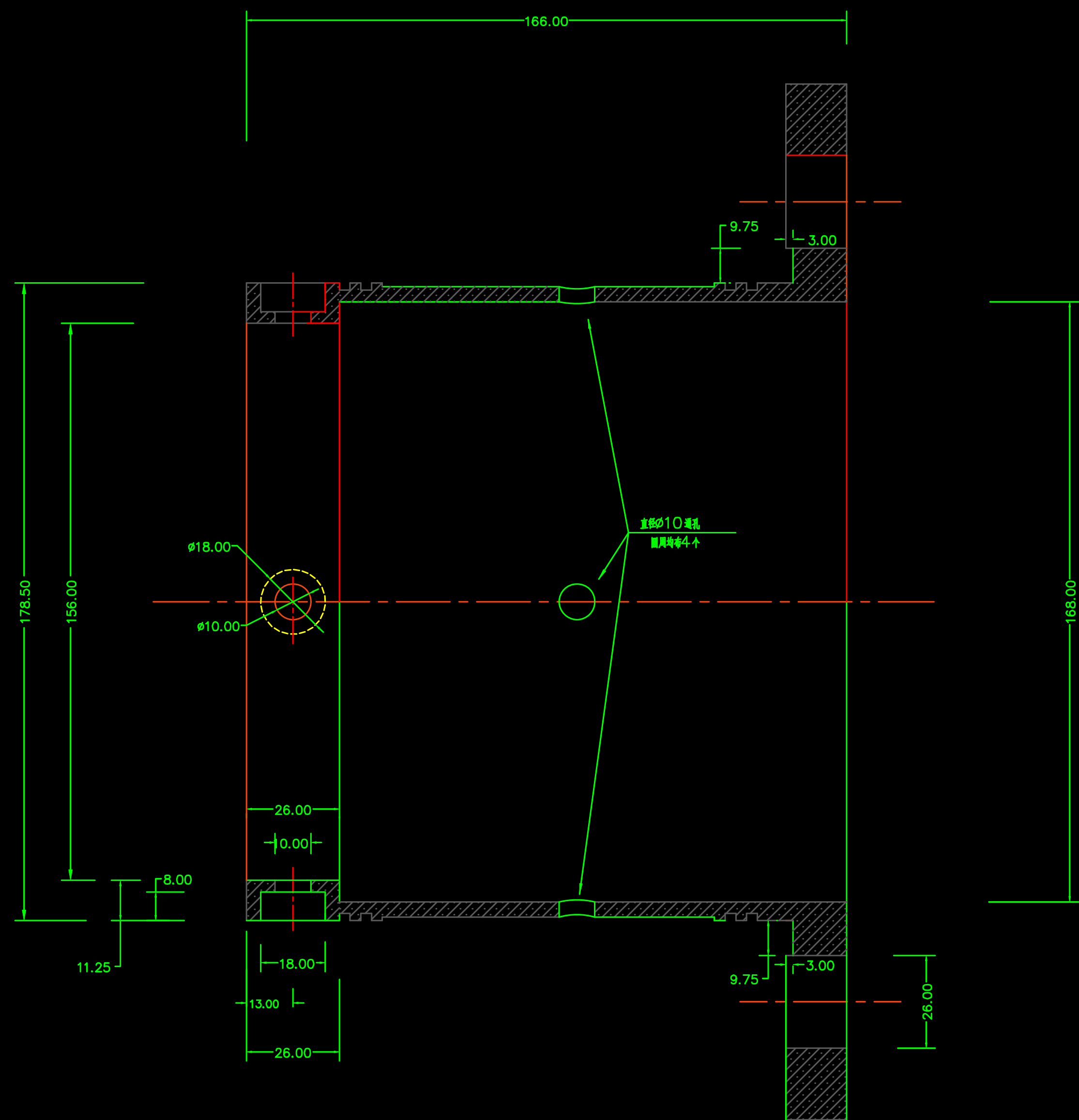
正视图
