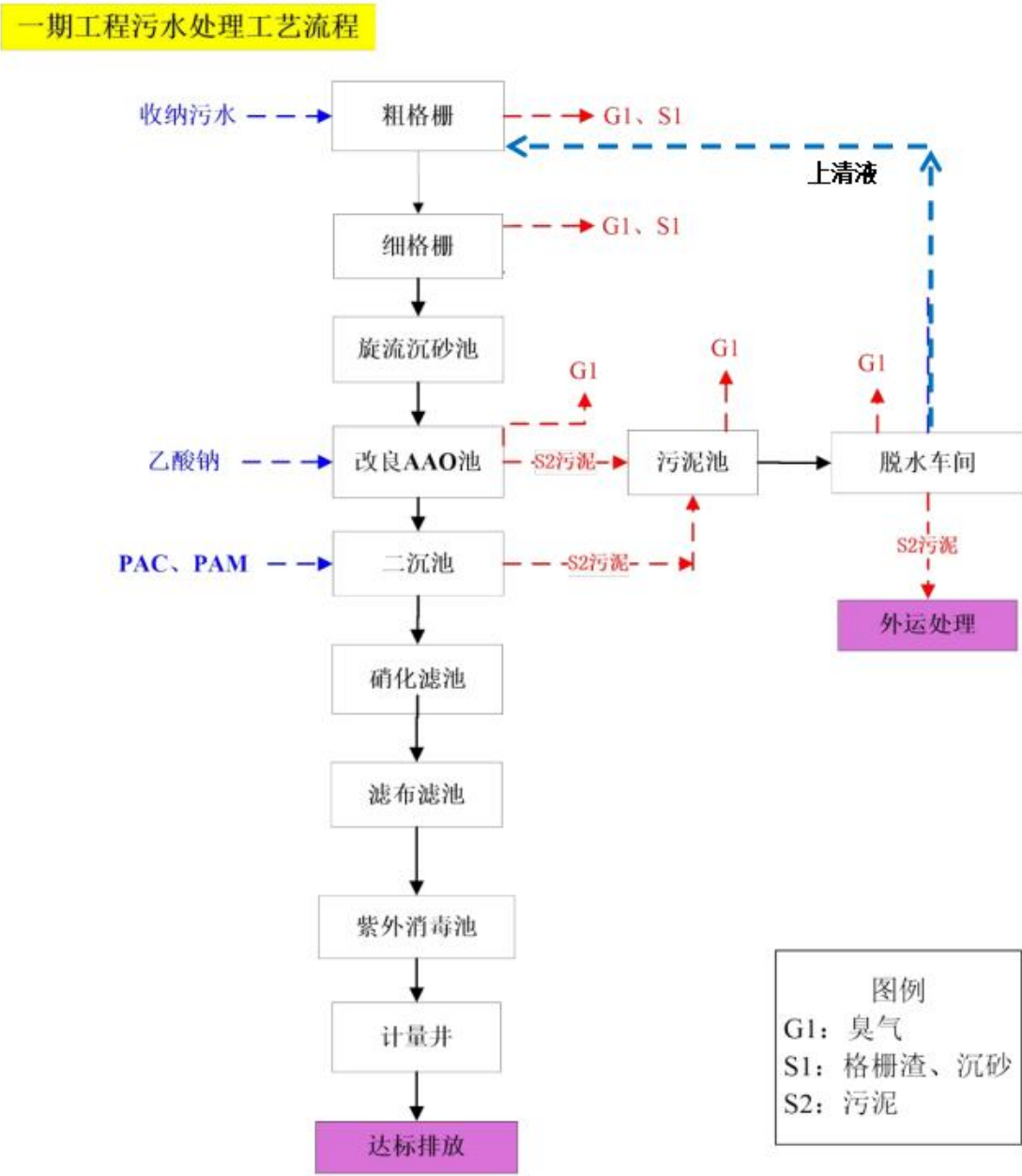
附图 11：污水处理工艺流程图
