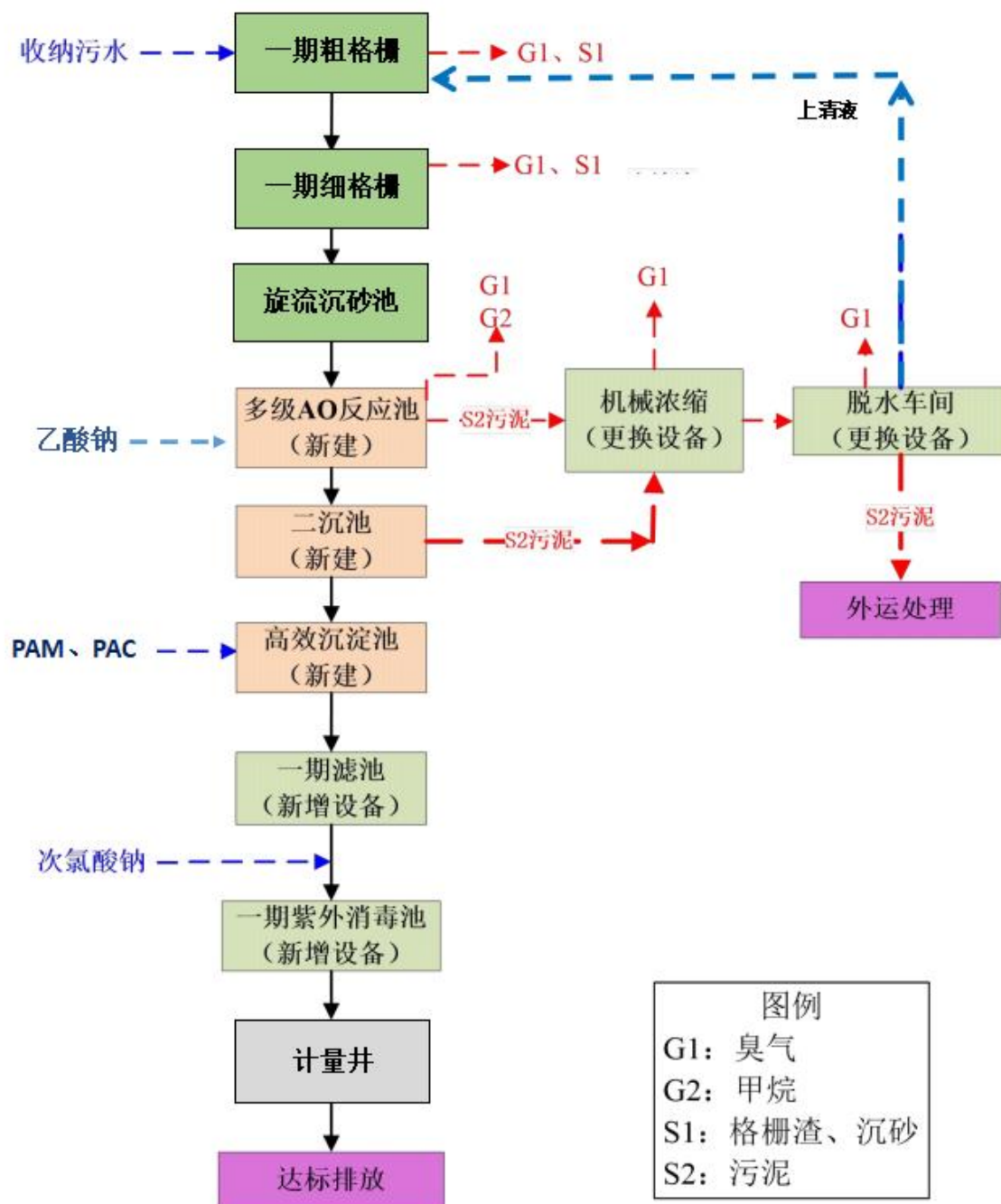
污水处理工艺流程图
