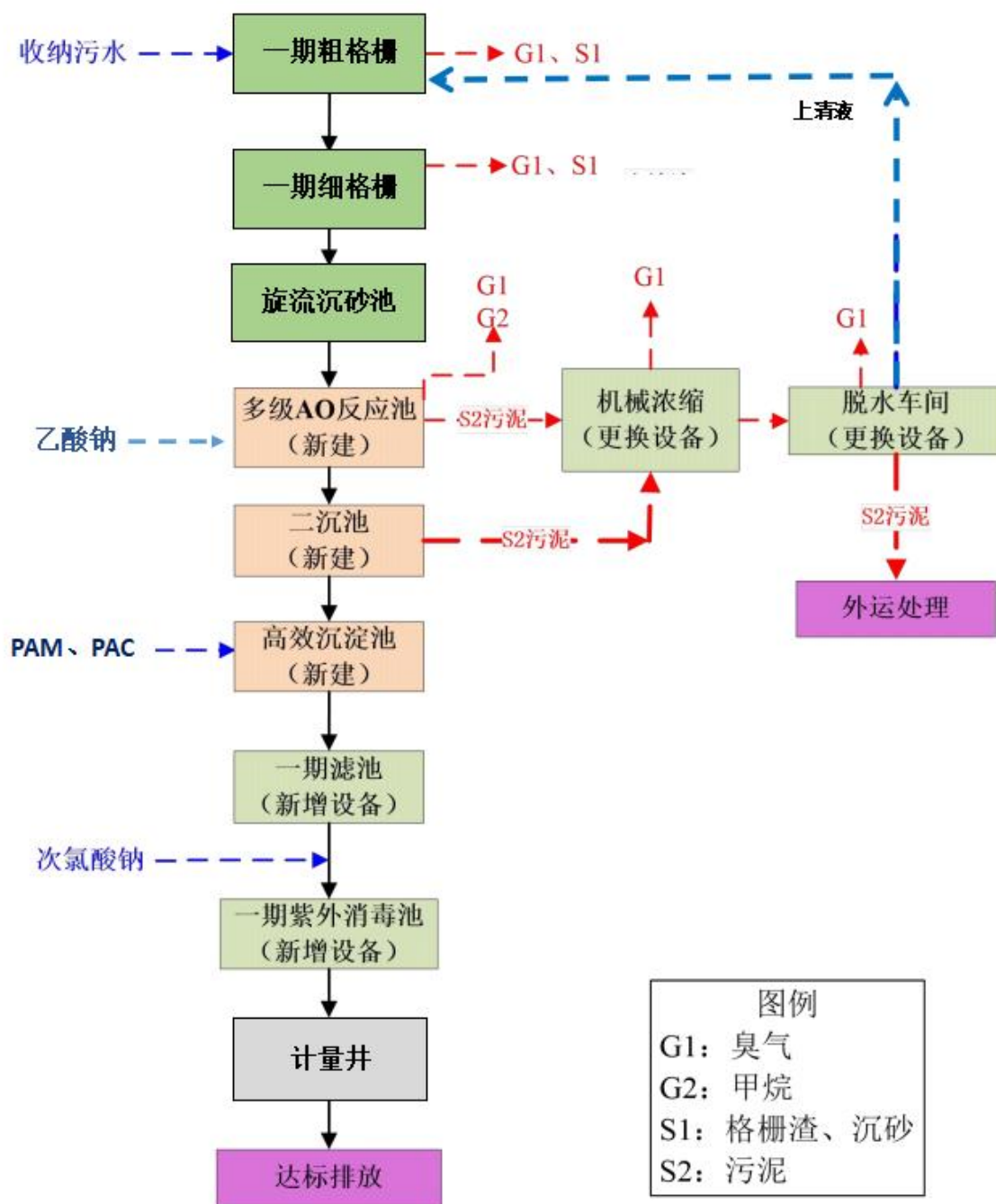
图 3.4-2 二期工程污水处理工艺流程图
