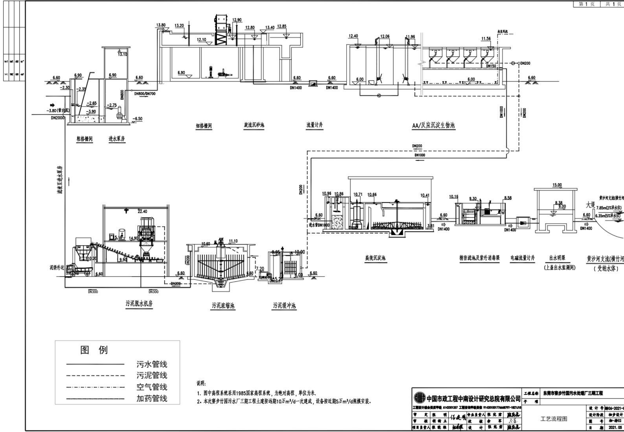
附图 12 项目工艺流程设备连接图
