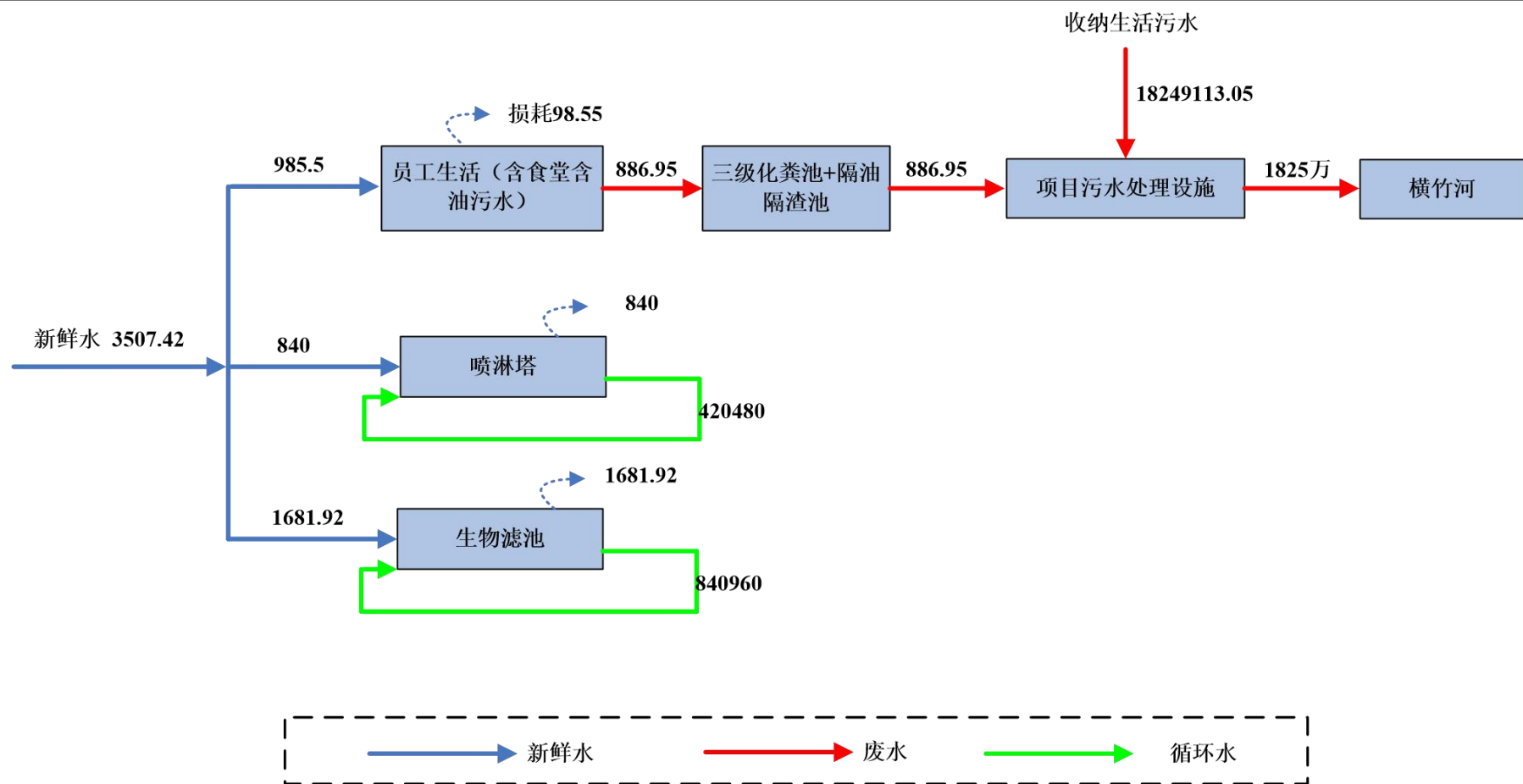
图 2-1 三期工程水平衡图 (单位: t/a)
