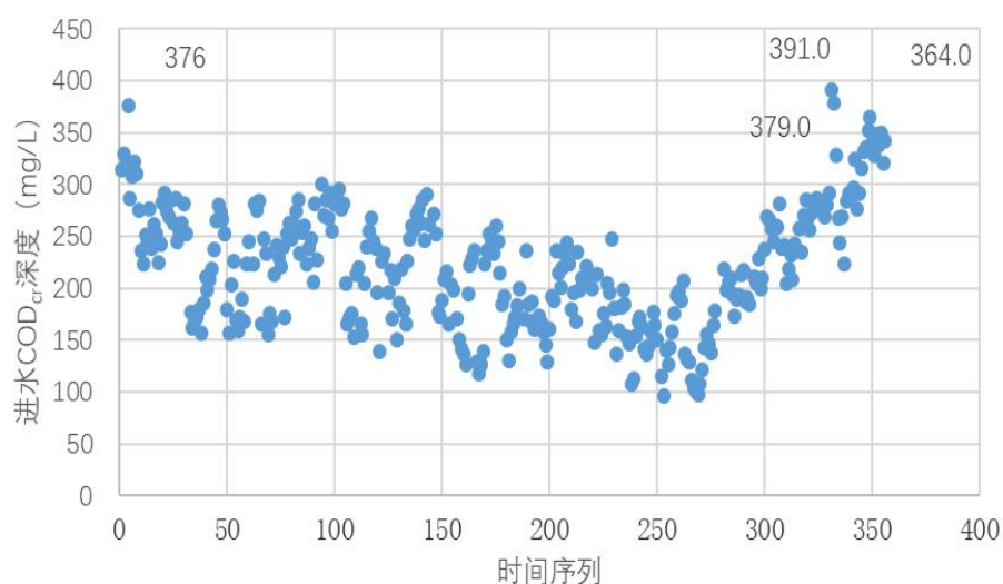
图 3.4-1 一期二期实测进水 COD Cr 统计散点图
