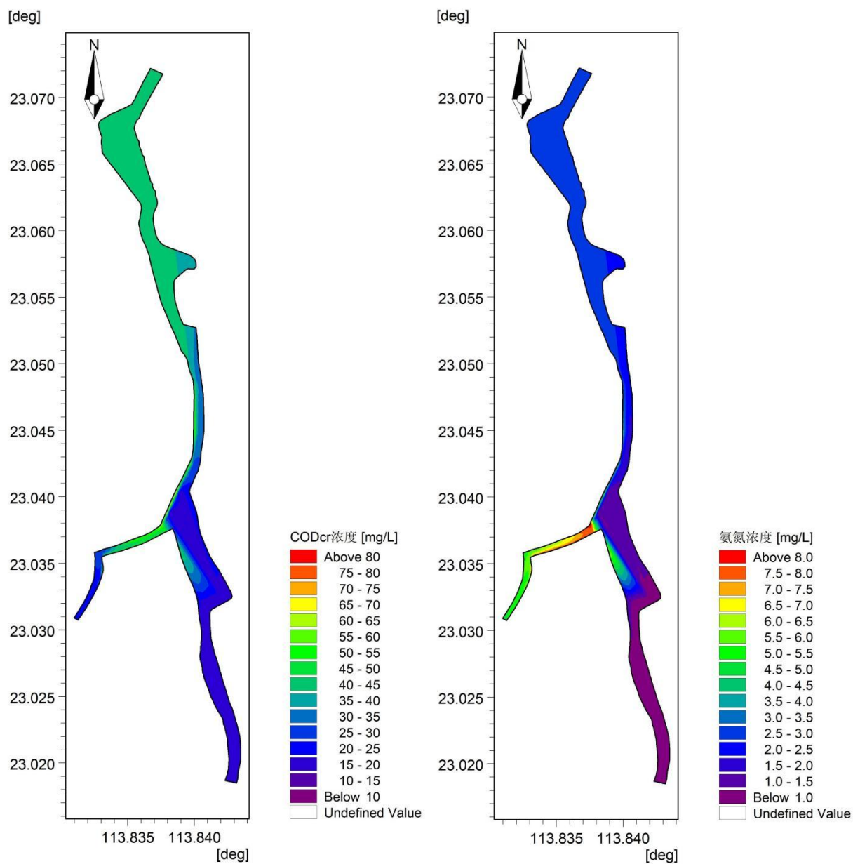
图 5.2-6a 枯水期情景一（本扩建工程和东城温塘水处理厂二期工程如未实施）
