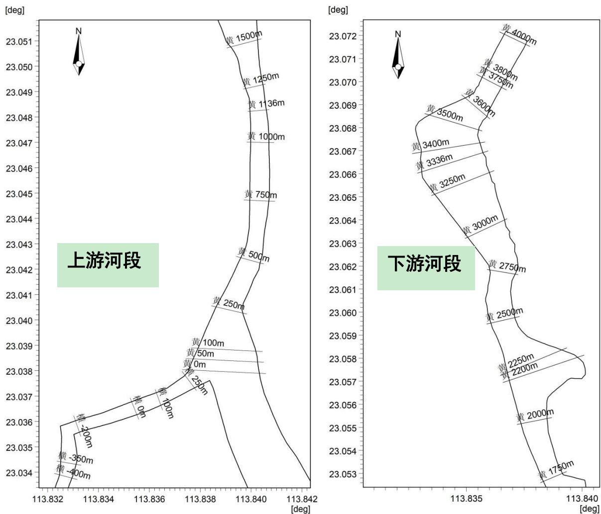
图 5.2-6 水质采样断面示意图
