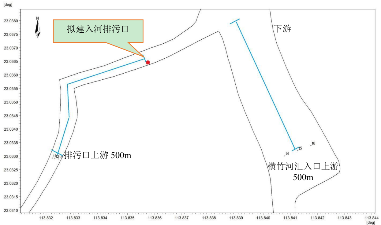
图 5.2-4 数学模型验证点位布置图
