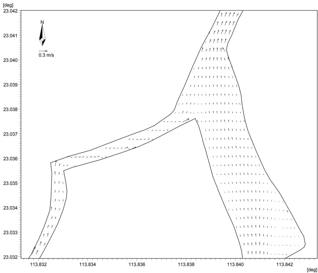
图 5.2-5a 枯水期工程局部流场图
