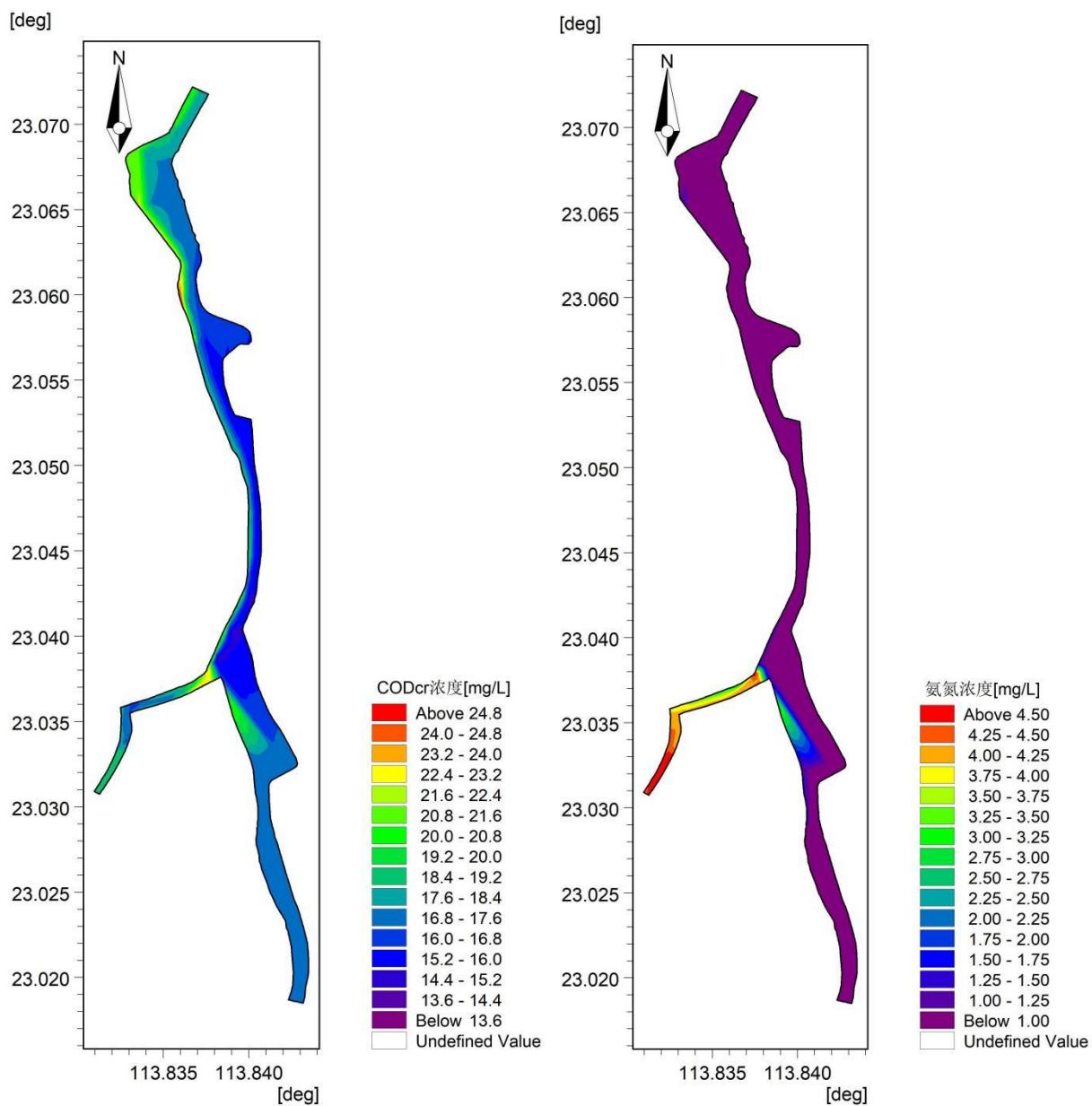
图 5.2-7b 丰水期情景二（本扩建工程和寮步竹园污水处理厂三期工程建设完成后，正常运行）
