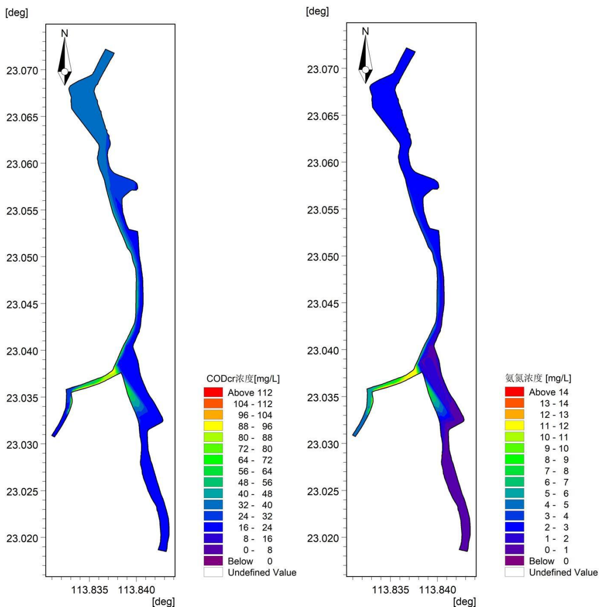
图 5.2-7c 丰水期情景三（本扩建工程和寮步竹园污水处理厂三期工程建设完成后，非正常运行）
