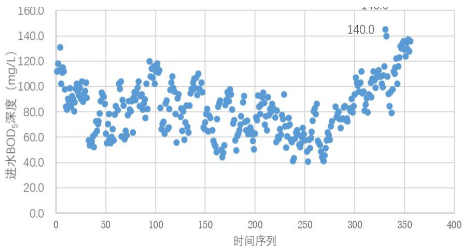
图 3.4-2 一期二期实测进水 BOD 5 统计散点图
