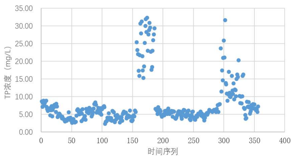
图 3.4-5 一期二期实测进水 TP 统计散点图
