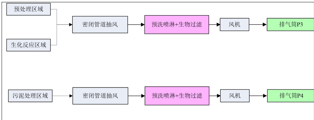
图 4-1 恶臭污染物治理工艺流程图
