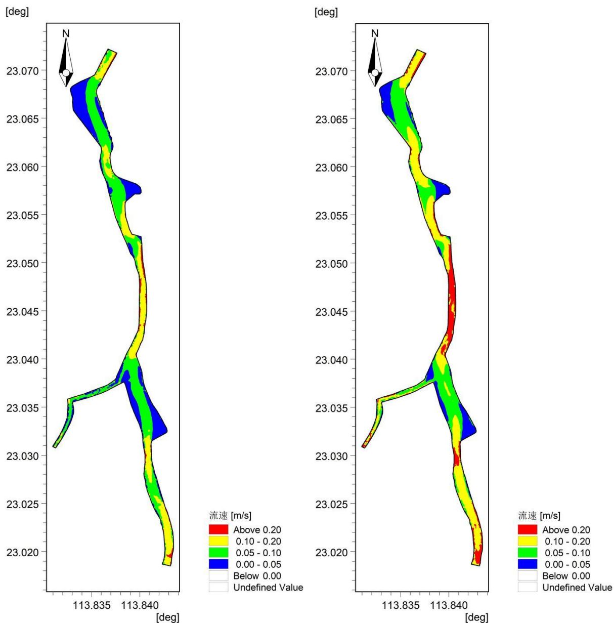
图 5.2-5c 枯水期、丰水期流速等值线图
