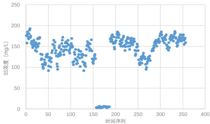
图 3.4-6 一期二期实测进水 SS 统计散点图
