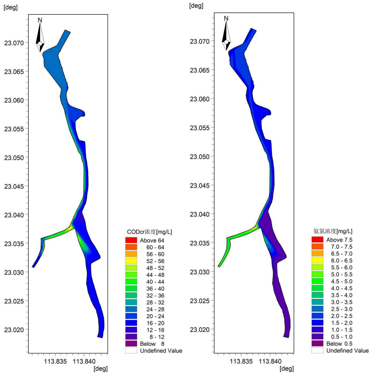
图 5.2-7a 丰水期情景一（本扩建工程和东城温塘水处理厂二期工程如未实施）
