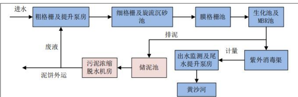
图 2-5 污水处理厂二期处理工艺流程
