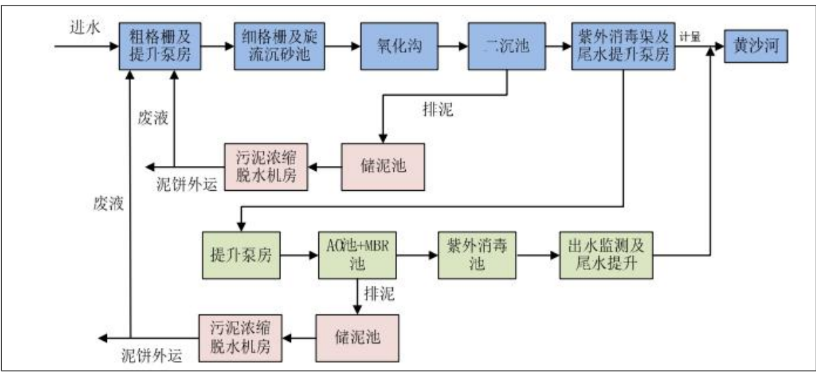
图 2-4 污水处理厂一期处理工艺流程
