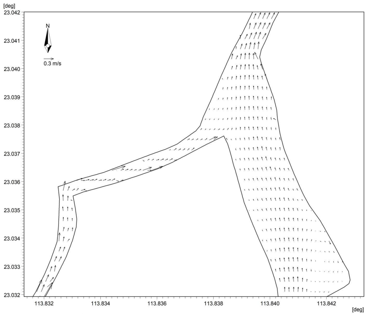
图 5.2-5b 丰水期工程局部流场图
