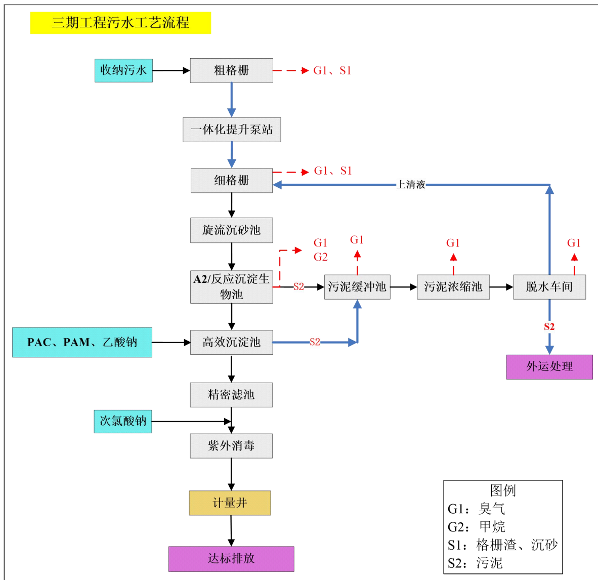
图 2-3 拟建项目运营期工艺流程图
