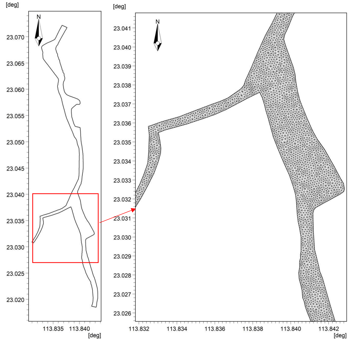
图 5.2-3 工程范围计算网格示意图
