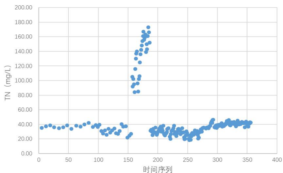
图 3.4-4 一期二期实测进水 TN 统计散点图
