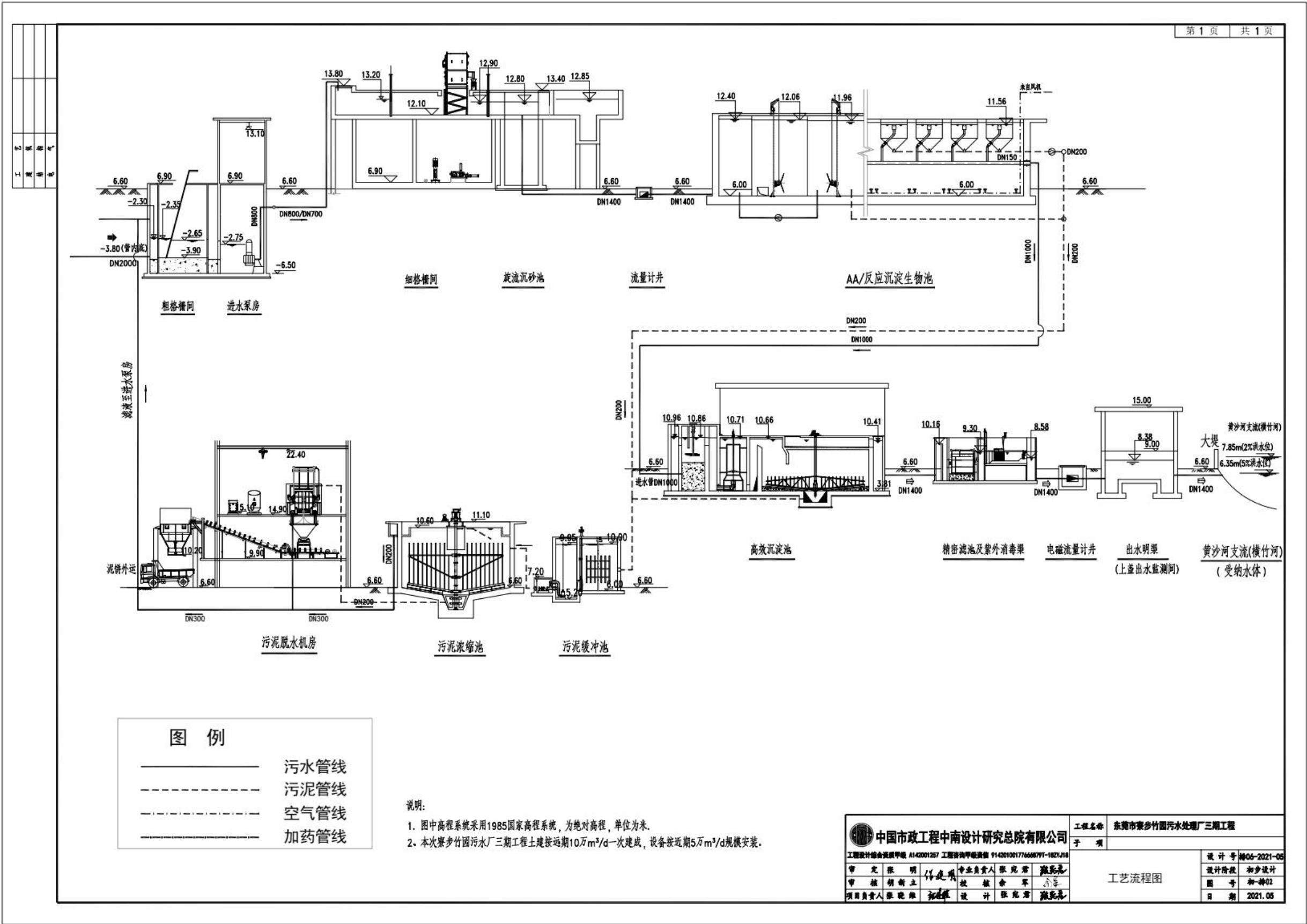
图 3.6-3 项目工艺设备连接图
