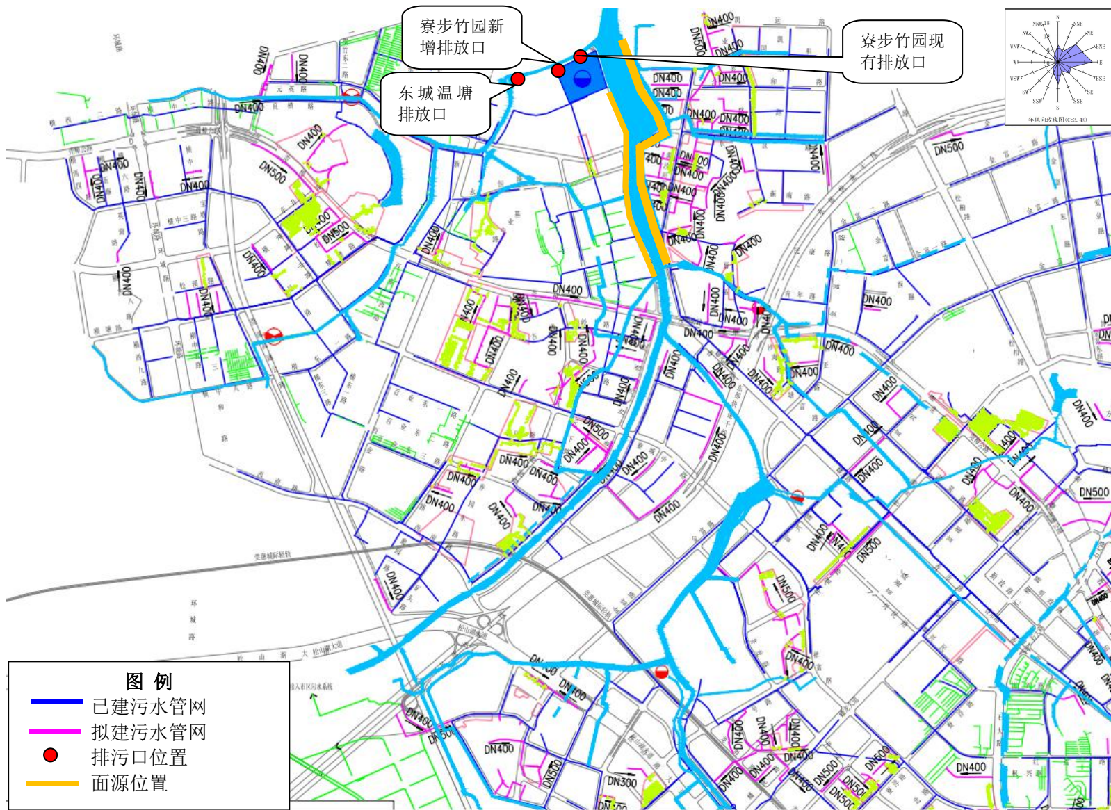
图 4.7-1 寮步镇拟建污染管网图 (节选)
