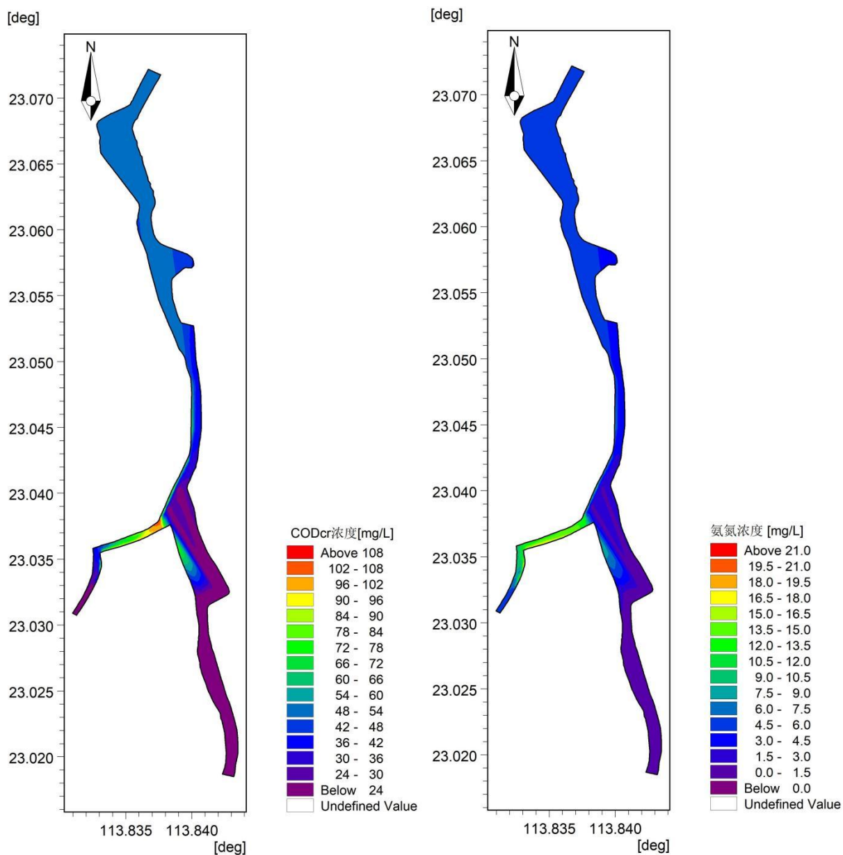
图 5.2-6c 枯水期情景三（本扩建工程和寮步竹园污水处理厂三期工程建设完成后，非正常运行）
