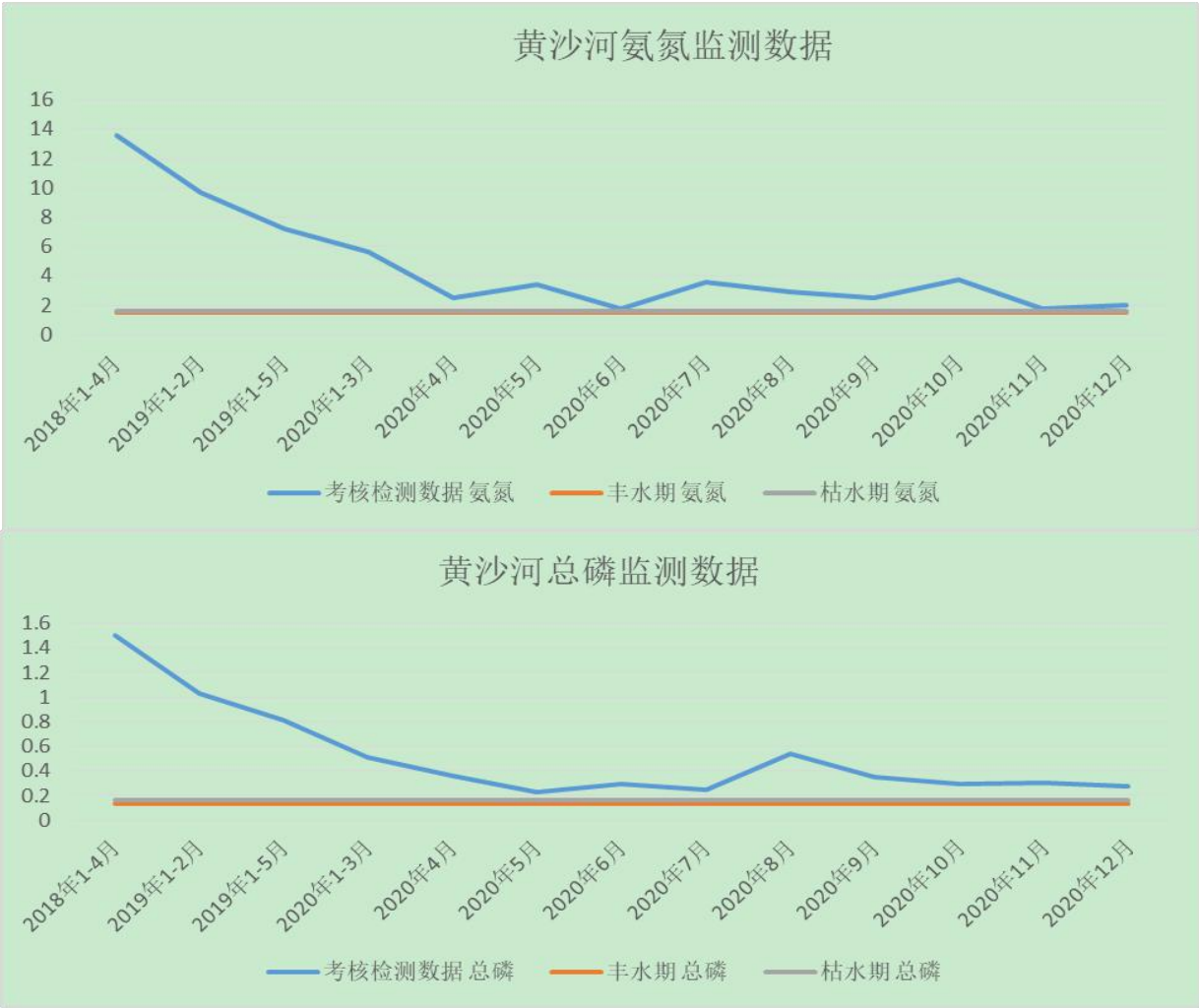
图 4.8-1 黄沙河水质变化趋势图
