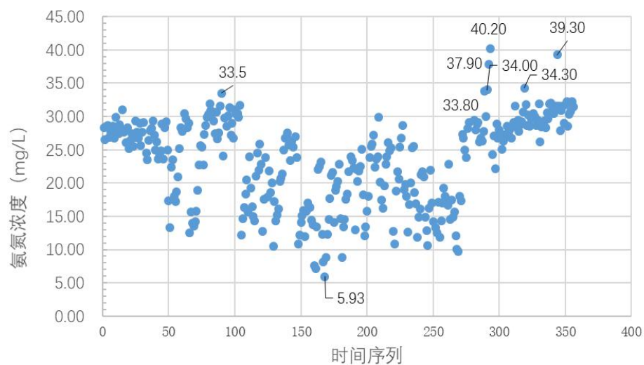
图 3.4-3 一期二期实测进水 \text{NH}_3\text{-N} 统计散点图
