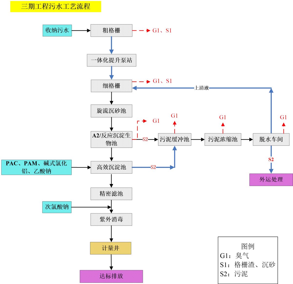
图 3.6-1 本项目运营期工艺流程图
