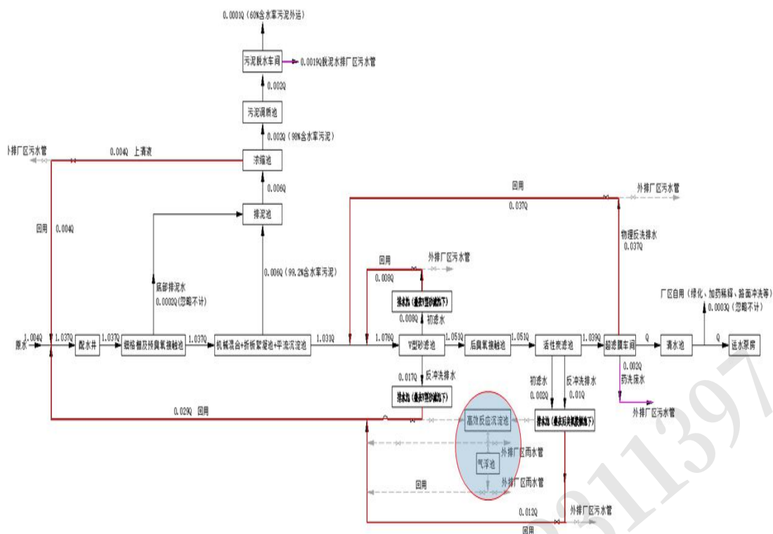
图 2 生产废水处理流程图
