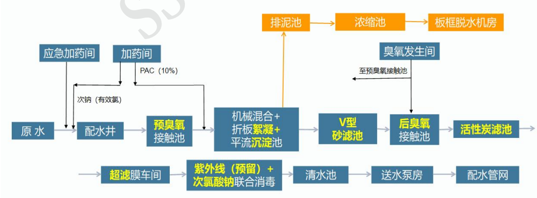
图 1 工艺流程图
