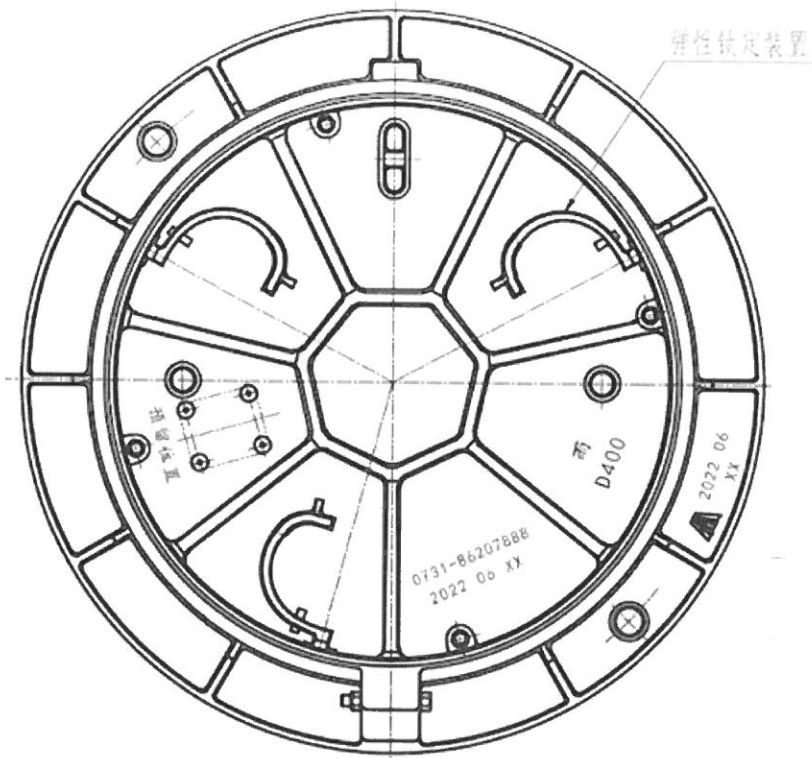
背面大样
