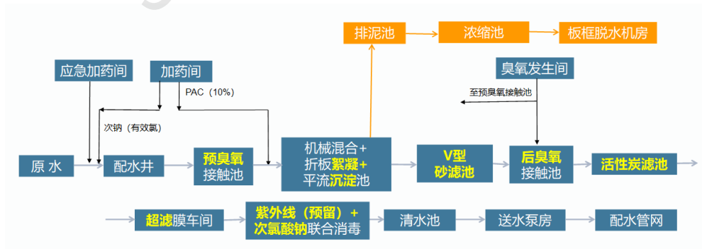
图 1 工艺流程图
