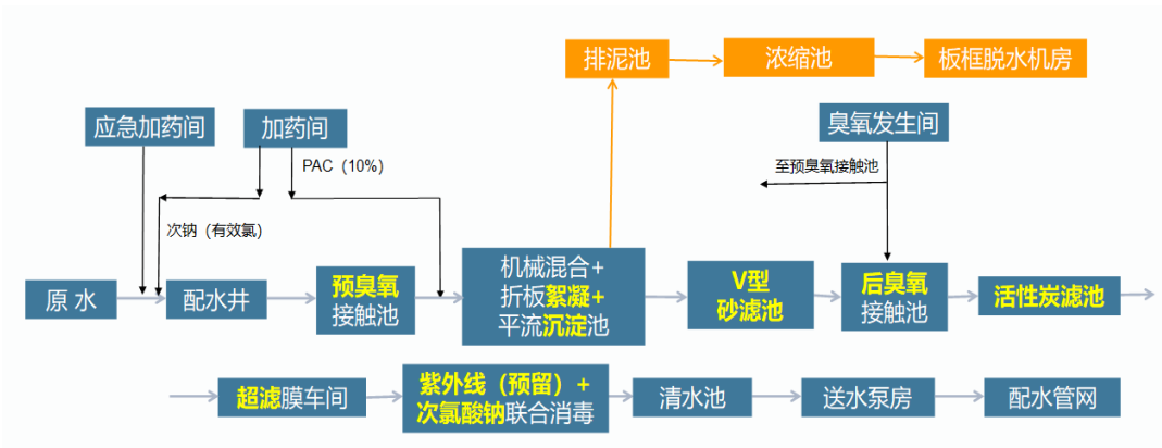
图 1 工艺流程图
