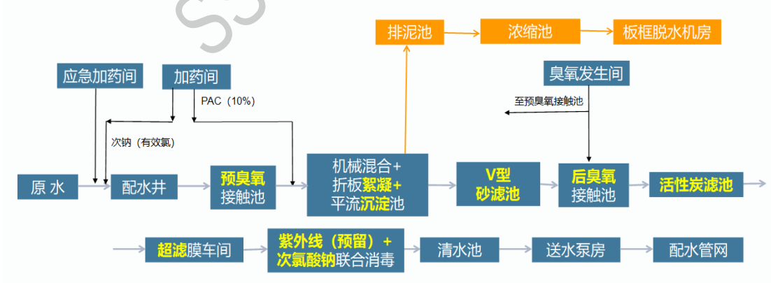
图 1 工艺流程图
