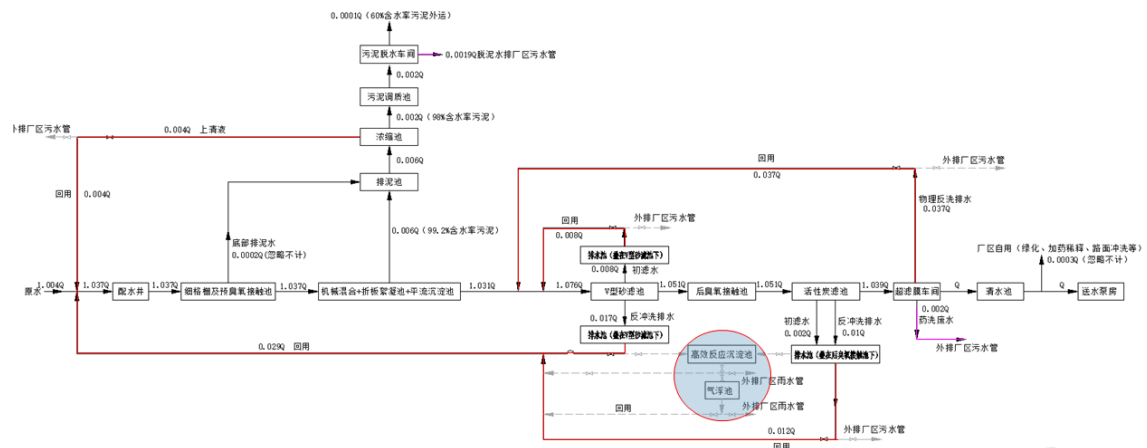
图 2 生产废水处理流程图
