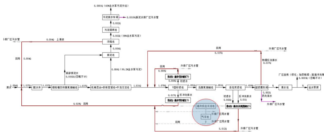
图 2 生产废水处理流程图
