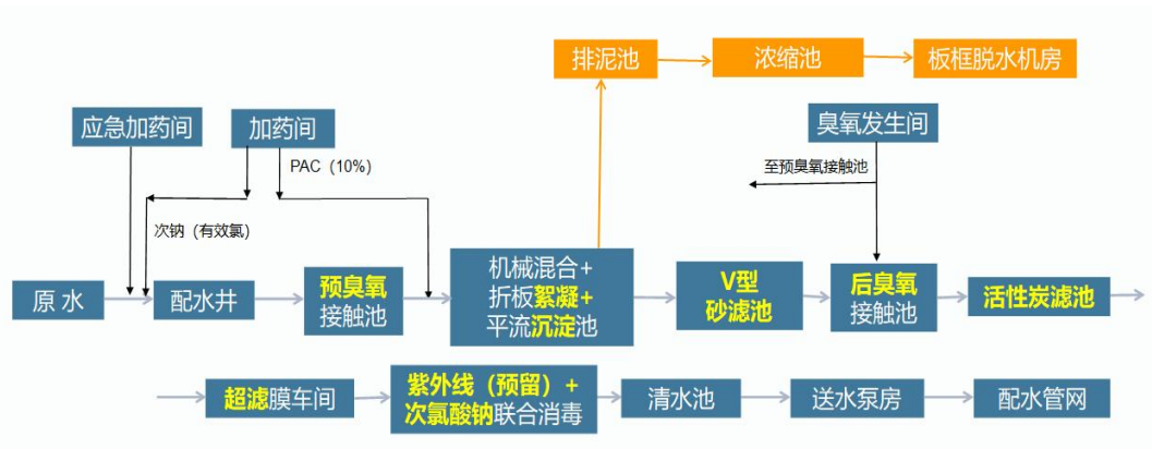
图 1 工艺流程图
