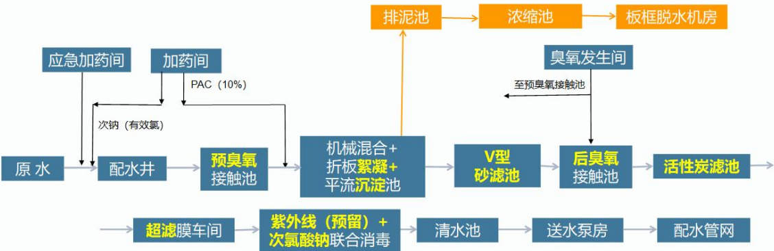
图 1 工艺流程图
