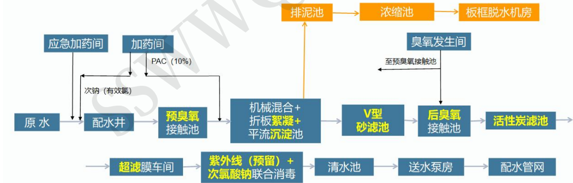
图 1 工艺流程图
