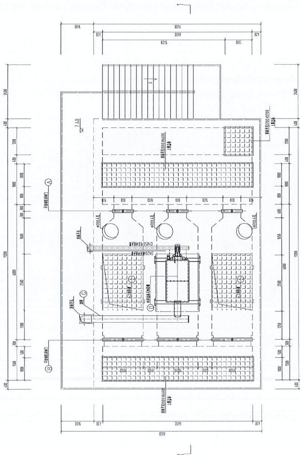
上层平面图 1:50
