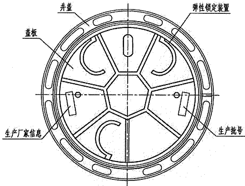
井盖设施底面平面图
