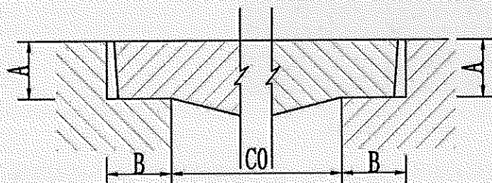
图 1：井座净开孔（C0）、嵌入深度（A）、支承面宽度（B） 图 2：总间隙 a=a_1+a_2
